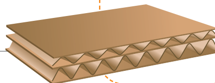
COUPE DOUBLE CANNELURE
